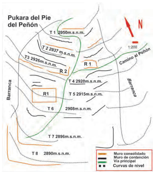
Fig. 11. Planimetría del Pukara del Pie del Peñón.
