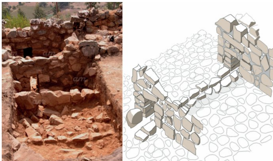
Foto e isométrico del sistema de ventilación/conservación de los productos almacenados en el silo de Incarracaycito en Pocona.
